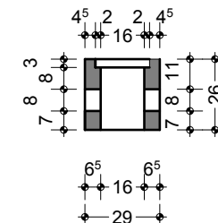
SEZIONE C-C SCALA 1:25
