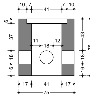
SEZIONE C-C SCALA 1:25
