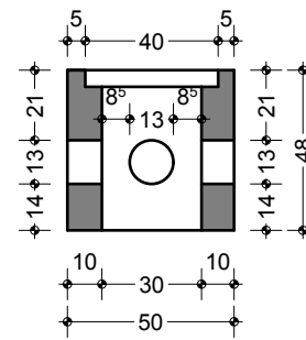
SEZIONE C-C SCALA 1:25
